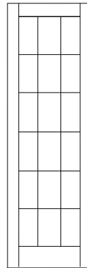
15 Lite (18) 8'0" Height 26", 28", 30", 32", 34", 36" widths
