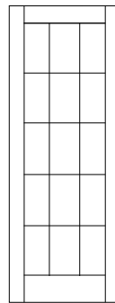
15 Lite 6'8" Height 26", 28", 30", 32", 34", 36" widths
